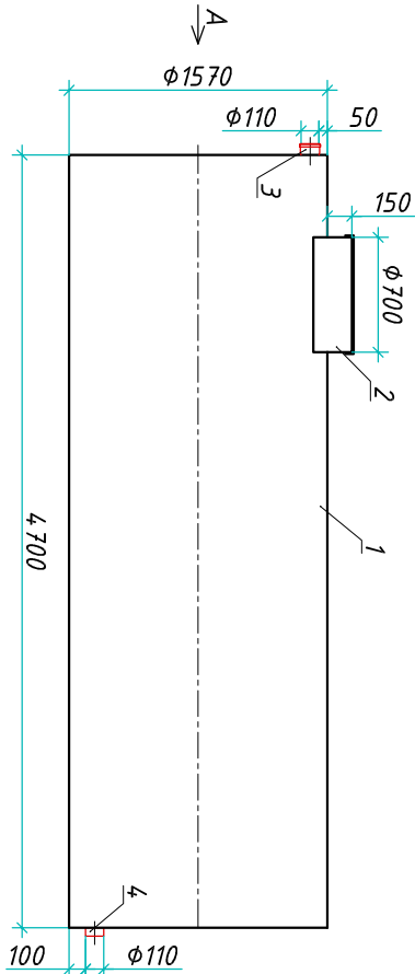
Разрез 1-1
