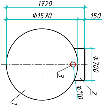
Вид А
