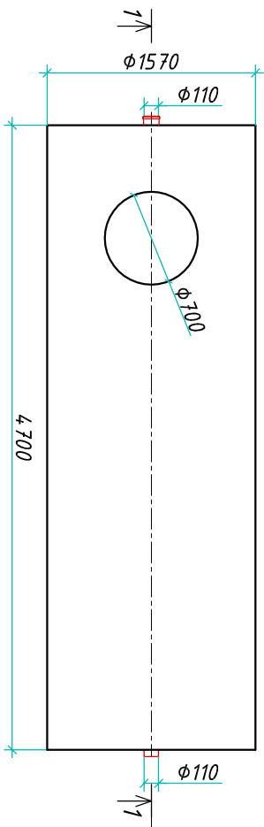
Вид сверху
